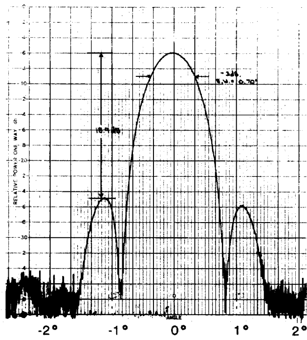
H-Plane — W-Band (12" Dia.)
